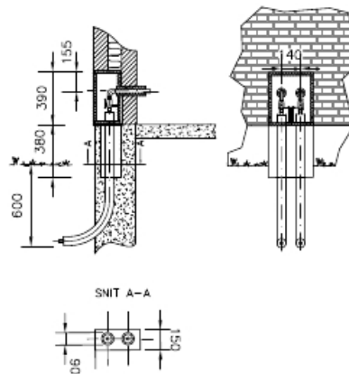
Figur 2 Tilkøbling med indføringsskab, indbygget i mur
