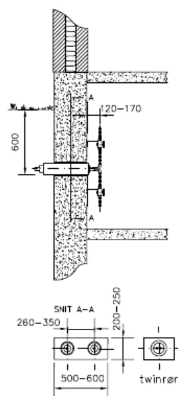
Figur 3 Lige gennemboring eller udsparring til bygning med kælder
