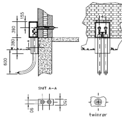
Figur 1 Tilkøbling med stikindføringsskab
